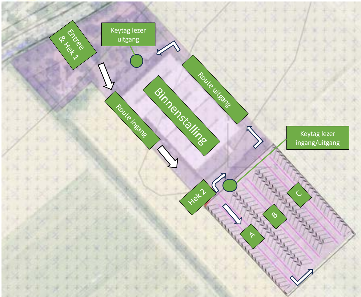
Afbeelding 3: Schematische weergave buitenstalling
